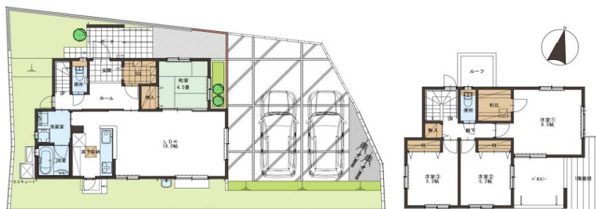
【間取り図】
